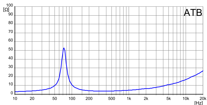
Impedanzverlauf / Impedance
